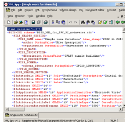
BLIS-XML document.
